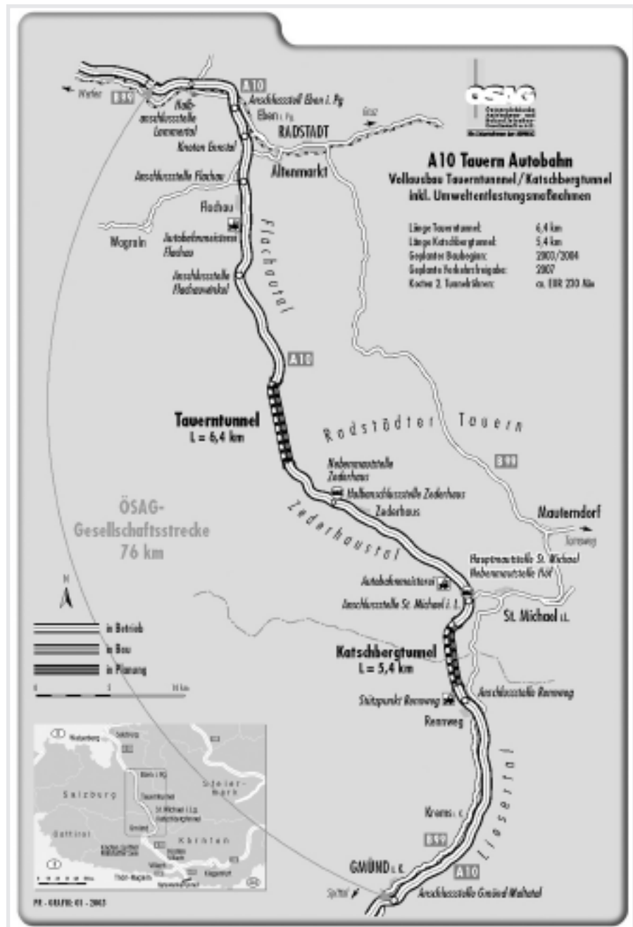
Abb. 1: Gesellschaftsstrecke der ÖSAG an der A 10 Tauern Autobahn
